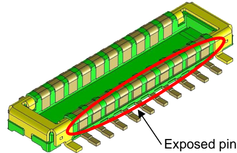
プラグ Plug PN: 505070-**20/-**40
