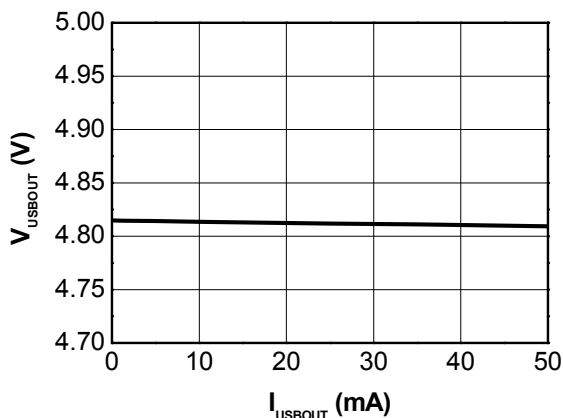
Figure 24. V_{USBOUT} vs I_{USBOUT} V_{USB}=5.0\text{ V} , T_A=25^\circ\text{C}
