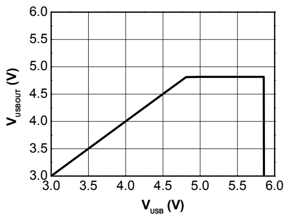
Figure 25. V_{USBOUT} vs V_{USB} I_{USBOUT}=0\text{ mA} , T_A=25^\circ\text{C}
